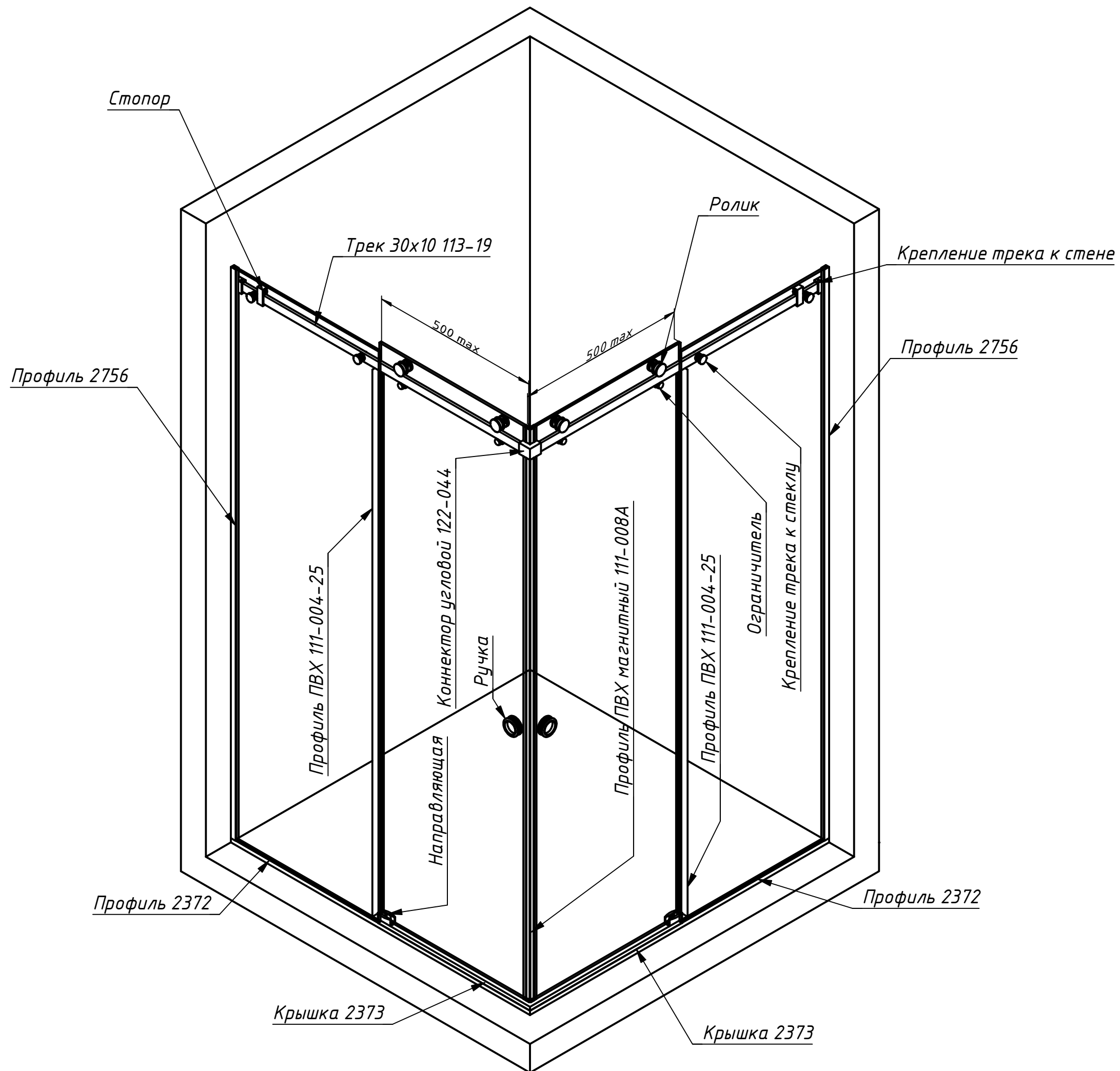
Схема угловой душевой кабины из 2-х комплектов 133-002
